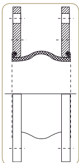
U Typ Standard kompensator för axiella, laterala och angulära rörelser.
