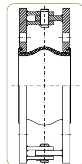
A Typ Utförande med hängslen för uppta- gande av angulära rörelser i ett plan.
