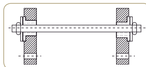
L1 Typ Gummibussningar för vibrationer
