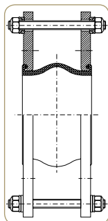
L Typ Kompensator med längdbegrän- sare för laterala rörelser.
