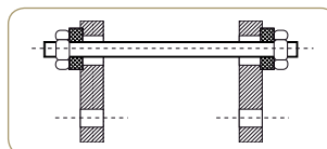
L2 Typ Sfäriska brickor för mjukare rörelser.
